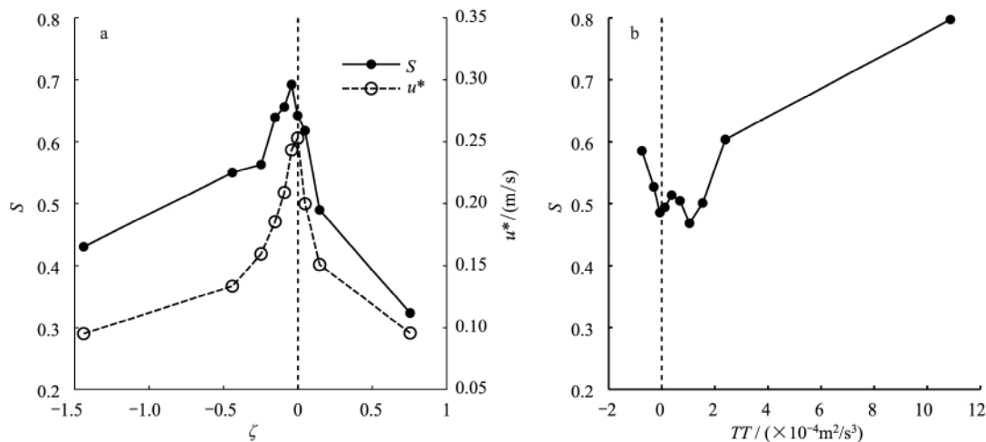
图7 BFG站能量闭合度 S 和摩擦风速 u^* 随大气稳定度参数 \zeta 的变化特征,能量闭合度 S 随热力湍流 TT 的变化特征
