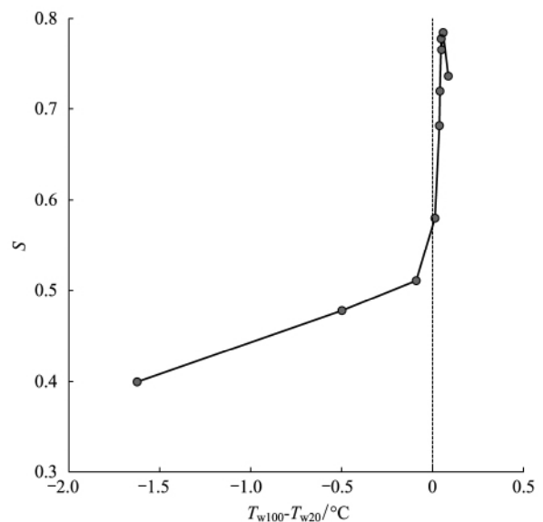
图 11 BFG 站能量闭合度 S 随水温梯度 ( T_{w100} - T_{w20} ) 的变化特征
