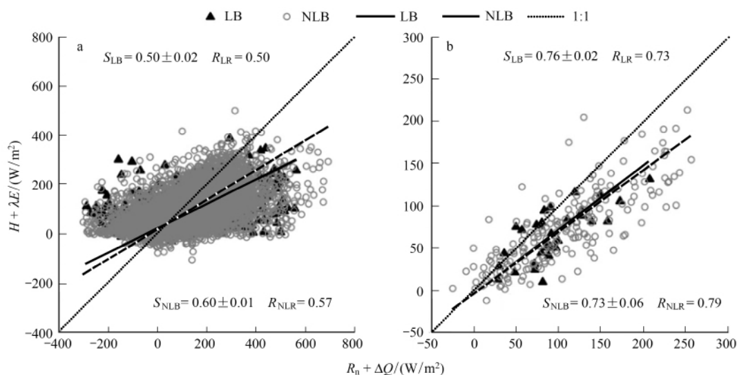
图 9 湖风发生(LB)及无湖风(NLB)时 BFG 站 (a) 半小时和 (b) 日平均湍流能量通量与可利用能量的线性回归关系
