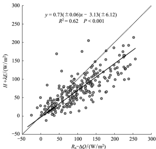
图5 2012年BFG站日平均湍流能量通量( H + \lambda E )与可利用能量( R_n - \Delta Q )的线性回归关系
