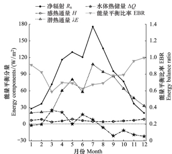
图6 2012年BFG站能量平衡分量和能量平衡比率(EBR)的季节变化特征
