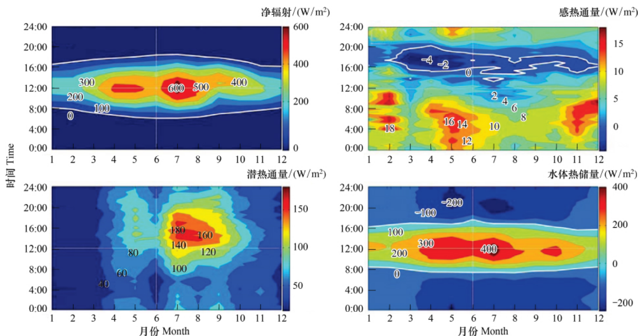
图 2 2012 年太湖 BFG 站能量平衡分量的月平均日变化( 改自 [49] )
