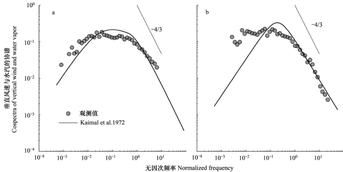
图 10 大气不稳定 (a) 和稳定条件下 BFG 站垂直风速与水汽密度的协谱 (b)
