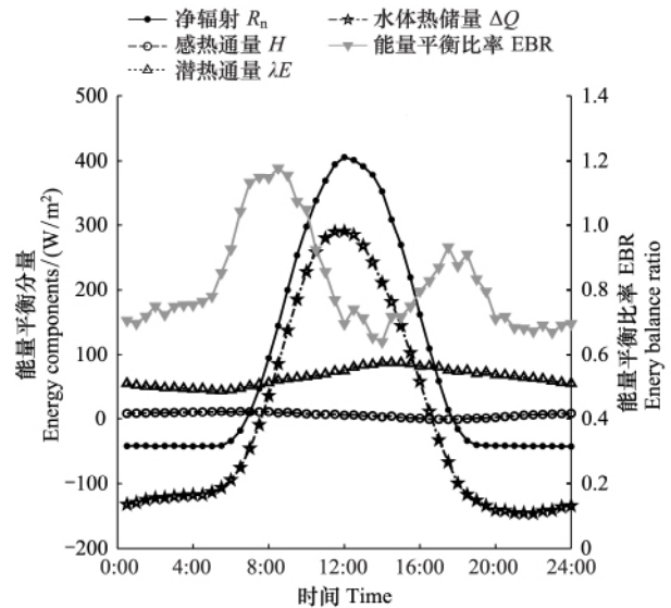
图 3 2012 年 BFG 站能量平衡分量和能量平衡比率(EBR)的年平均日变化
