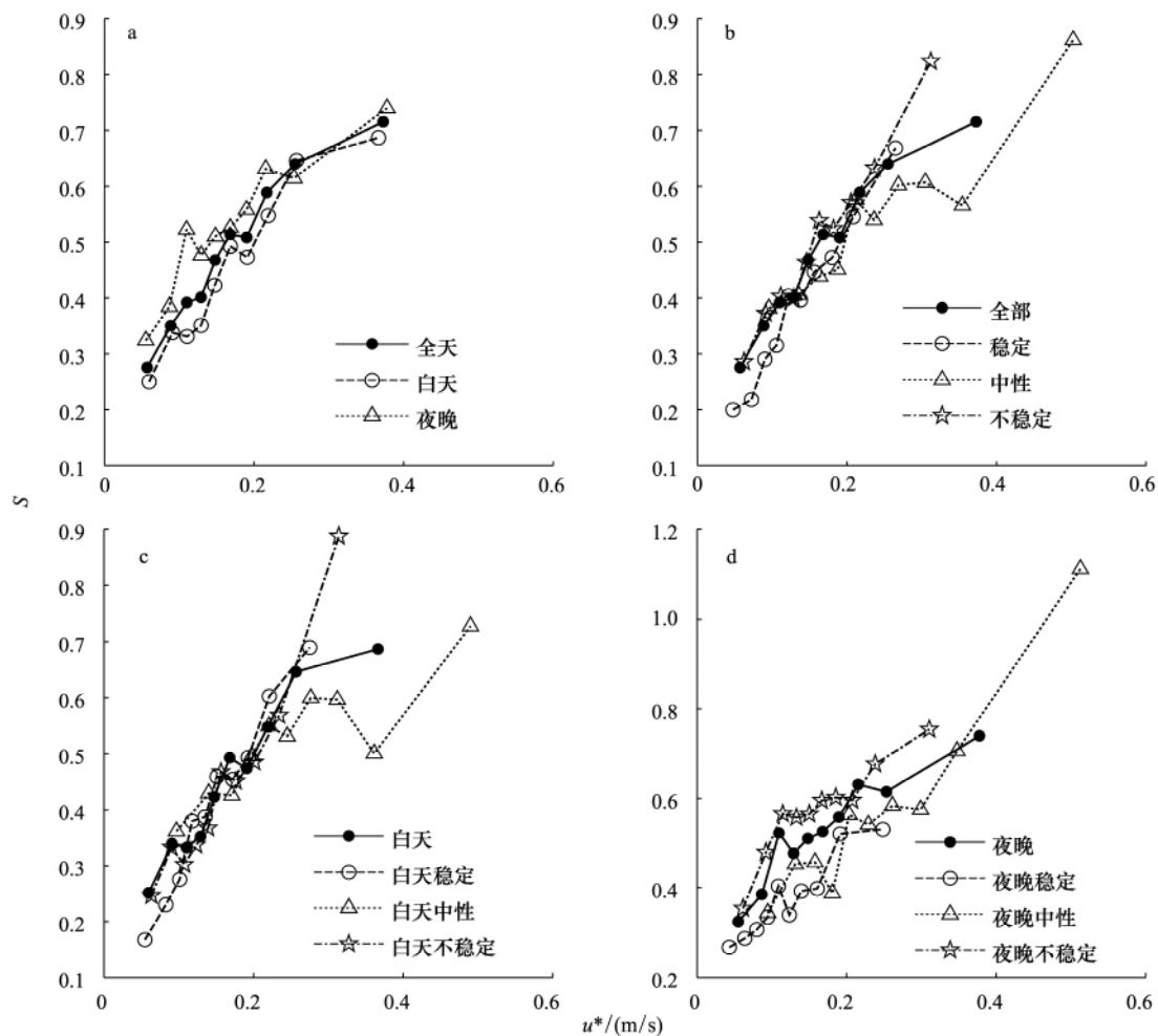
图 8 昼夜和不同大气稳定度下 BFG 站能量闭合度 S 随摩擦风速 u^* 的变化特征 [49]
