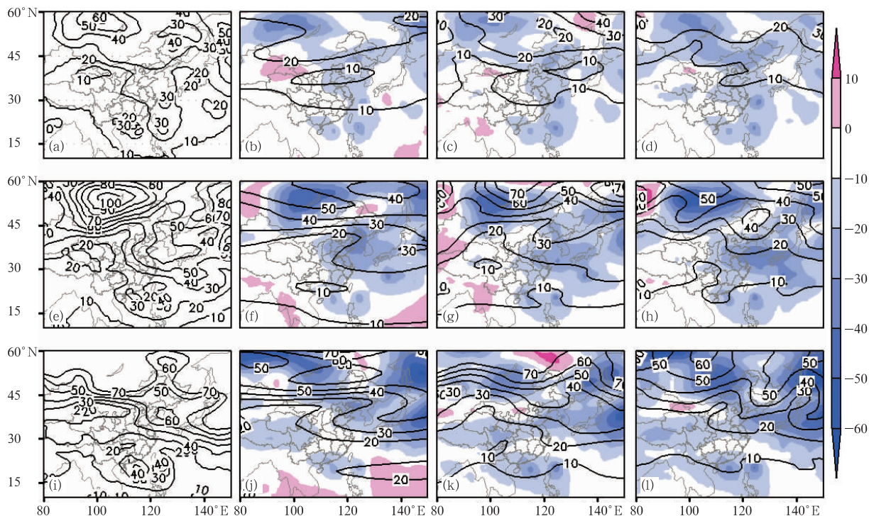
图3 2012年7月11—31日500 hPa位势高度场超长波(1~3波: b, f, j)、长波(3~6波: c, g, k和5~8波: d, h, l)的不同时效(5 d: a~d, 10 d: e~h和15 d: i~l)预报与分析场(a, e, i)的RMSE空间偏差分布
